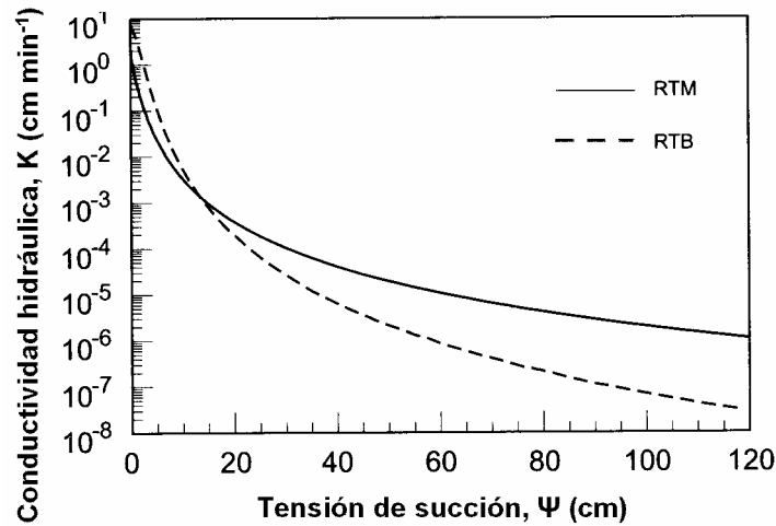
Figura 1. Conductividad hidráulica calculada versus tensión de succión, K(\psi) , para picón de los tipos RTB y RTM (Wallach y col, 1992; citado por Raviv y col, 2002)
